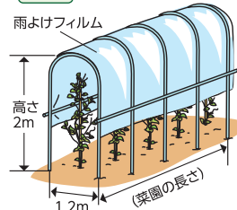
図3 雨よけ
